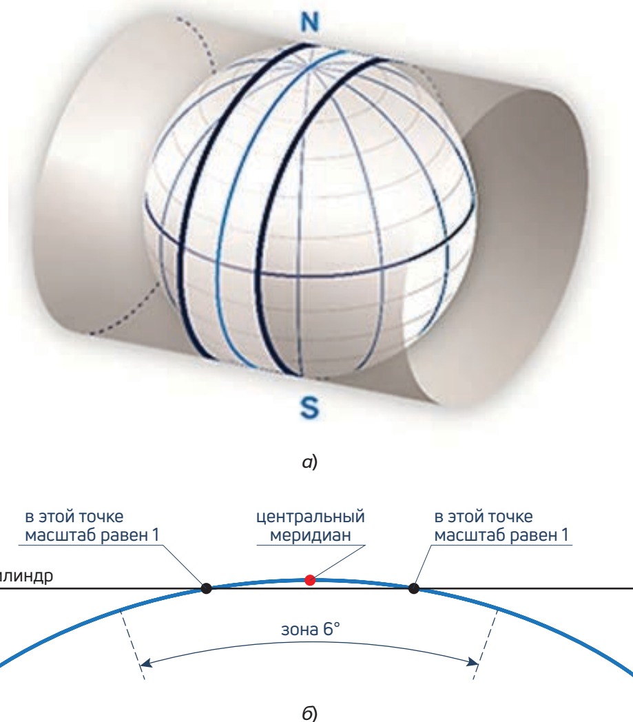
Рисунок 3. Универсальная поперечно-цилиндрическая проекция Меркатора
