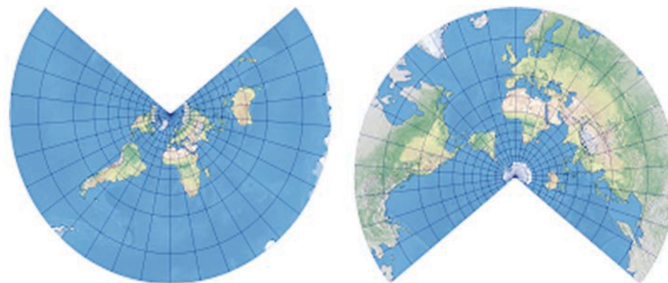
Рисунок 5. Равноугольная коническая проекция полушарий Ламберта
