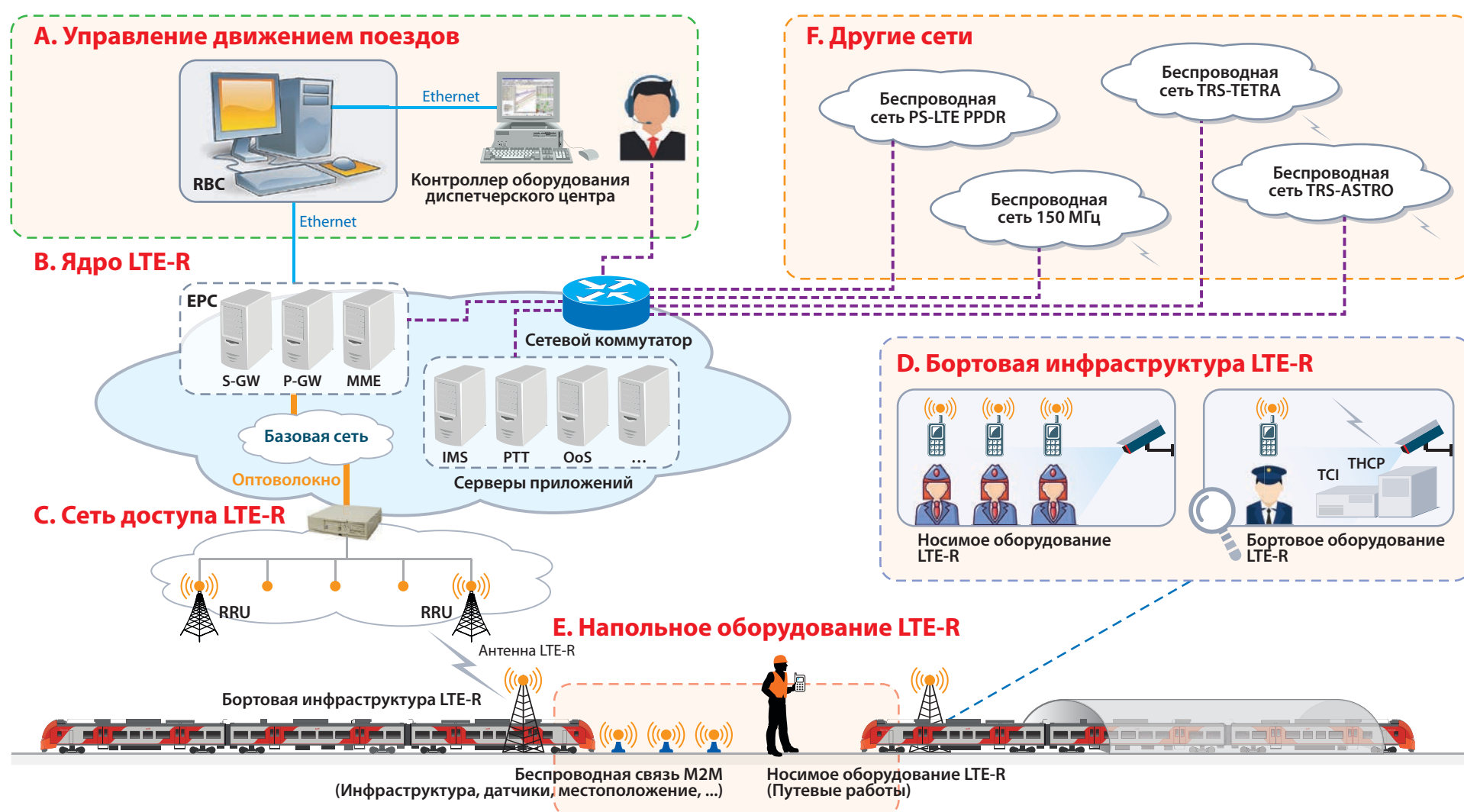
Рисунок 5. Структура перспективной системы технологической радиосвязи
