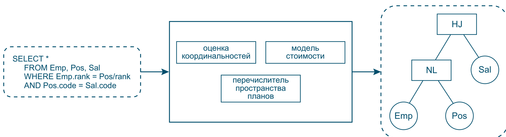
Рисунок 2. Архитектура традиционного оптимизатора запросов
